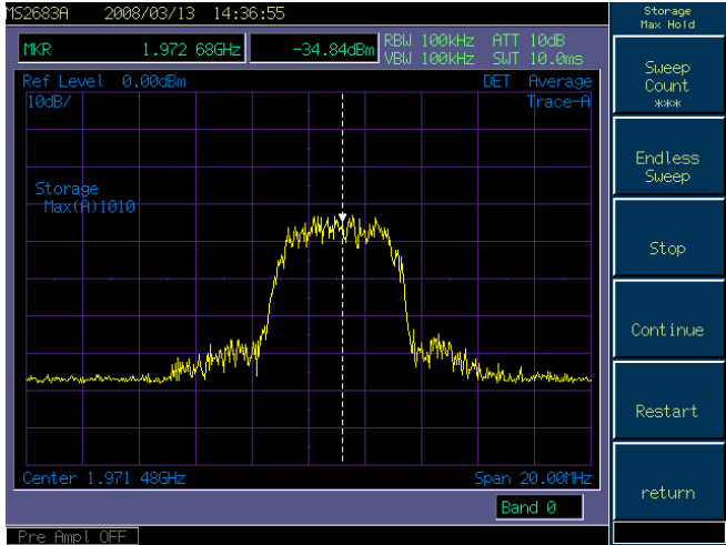
LOAを貼る前の波形
