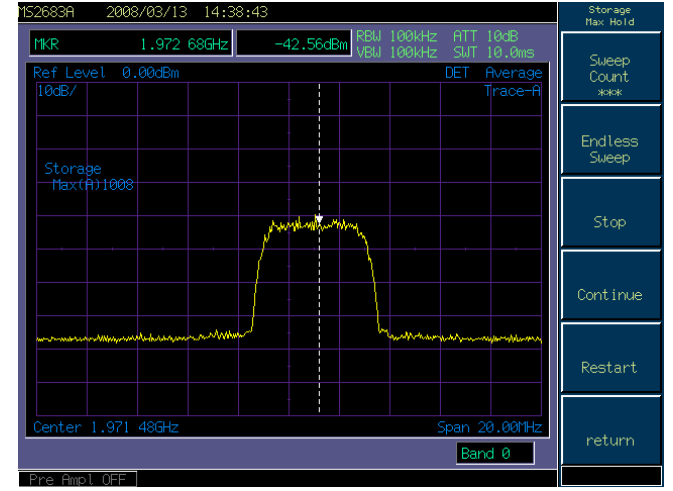
LOAを貼った後の波形
